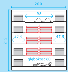
szafa DEN-20 (opcja z półkami)
