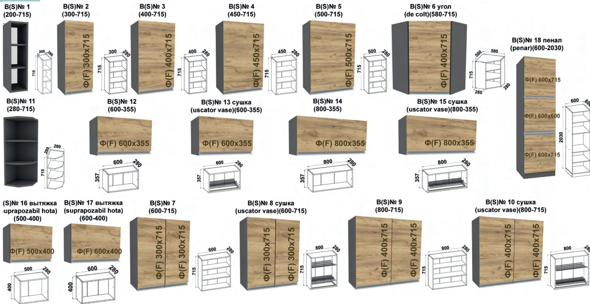
Inaltime carcasa superioara: 715 mm Adancime carcasa superioara: 280 mm
